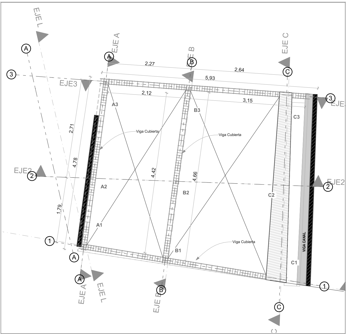
Planta de Cubierta +7.50 Esc 1: 50
