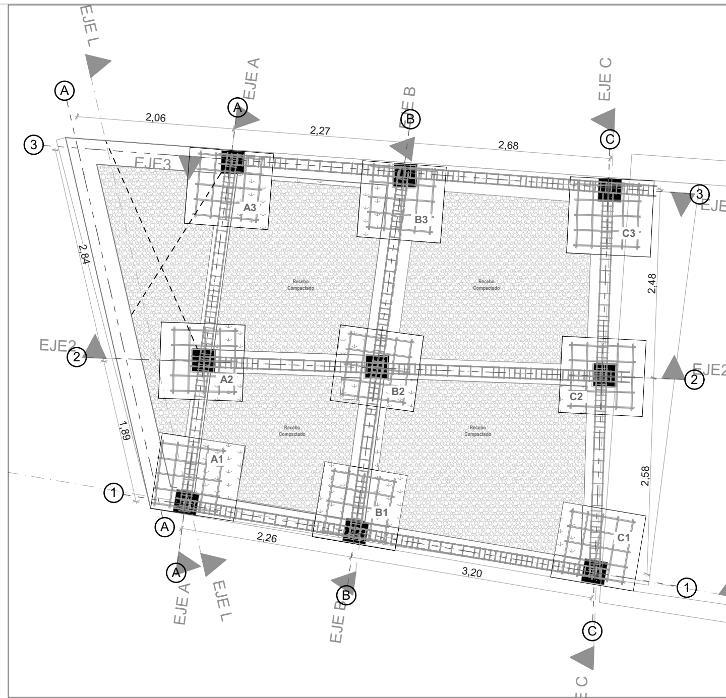
Planta de Cimentación +0.00 Esc 1: 50
