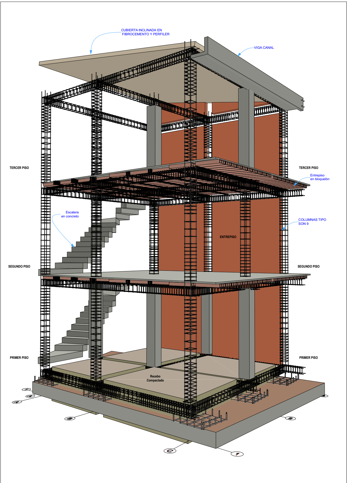
Vista del Proyecto Axonometría
