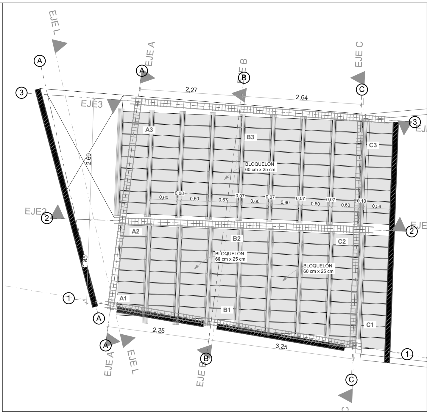
Planta tipo de Entrepiso +2.50 /+5.00 Esc 1: 50
